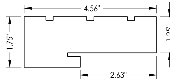
1 DOOR JAMB
