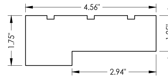
4 SIDELITE JAMB
