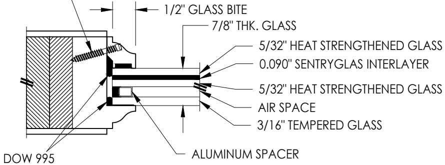
G2 GLAZING DETAIL
